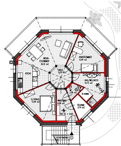
Außenansicht und Grundriss des MB-Haus Muster-Passivhauses am Sonnenplatz in Großschönau.
